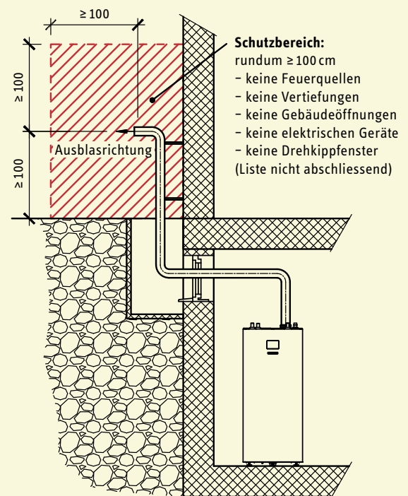
Erdsonden-Wärmepumpe WPE-I mit Entlüftungsvorkehrungen
